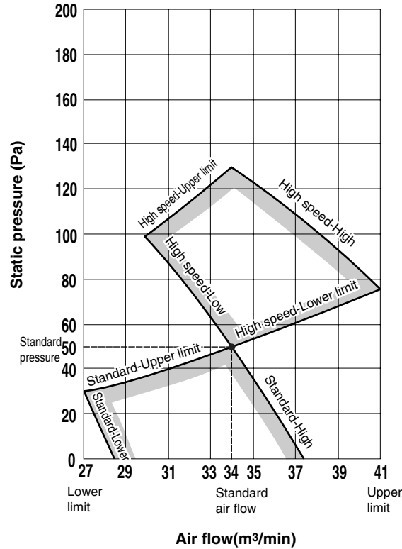
Model FDU112KXE6
