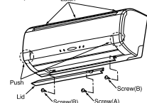
Fig.1(CASE1)
