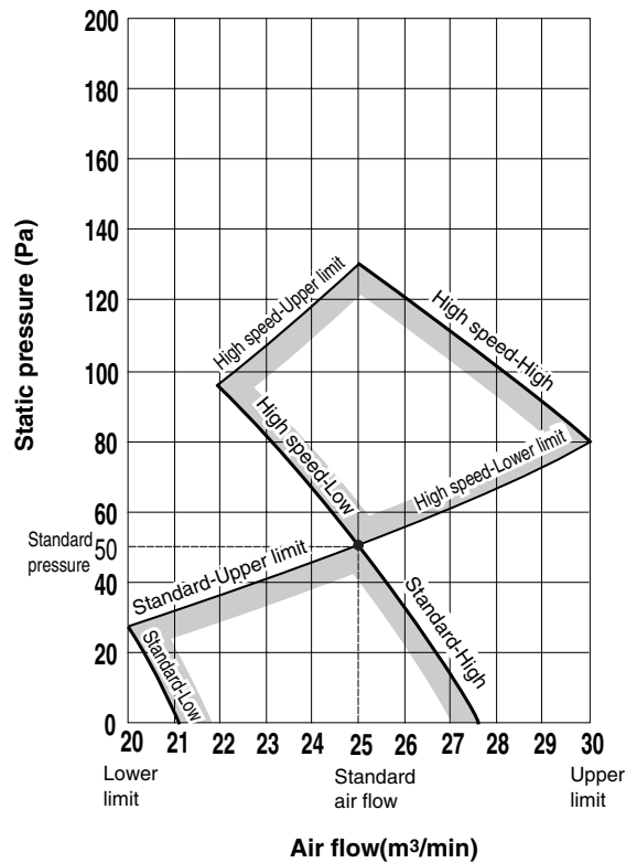
Model FDU71KXE6
