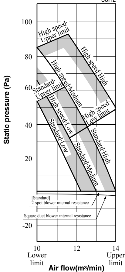
Models FDUM28KXE6,36KXE6
