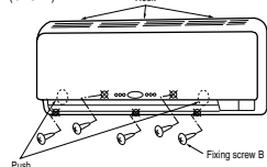
Fig.2(CASE2)
