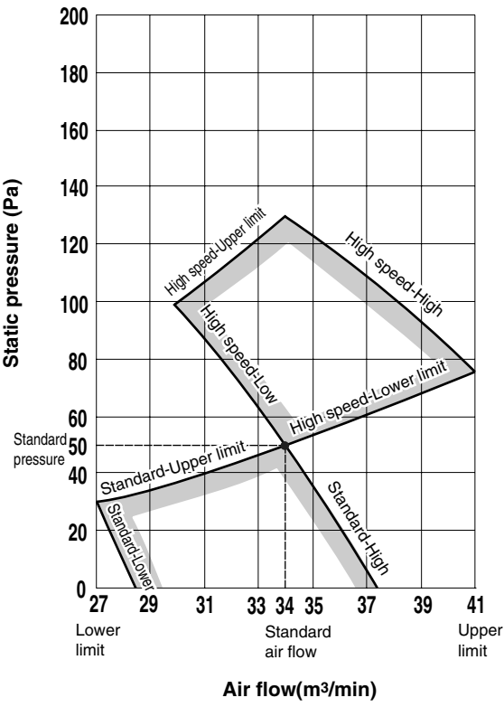
Model FDU90KXE6
